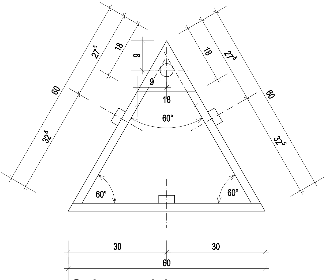
Seitenansicht
